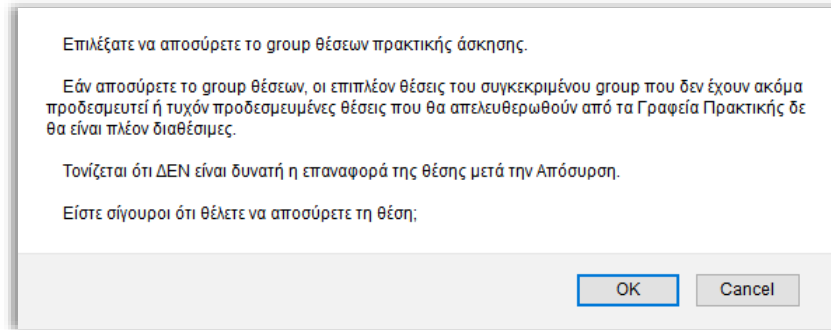
Εικόνα 3.6.3 – Επιβεβαίωση Απόσυρσης
