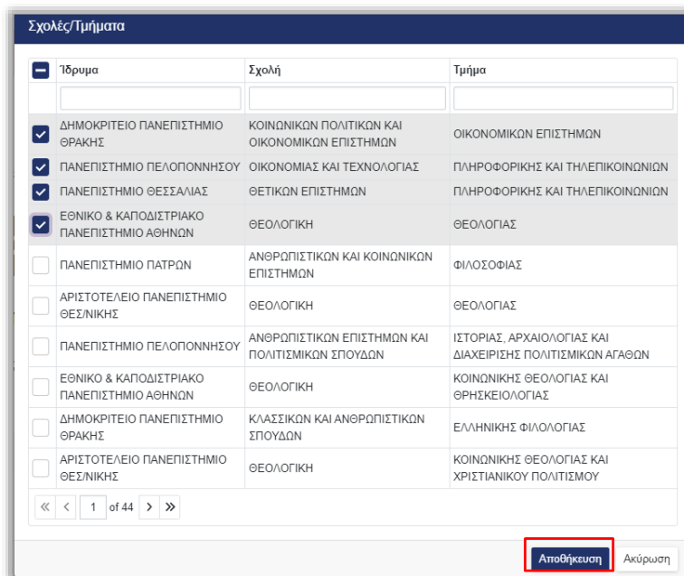
Εικόνα 3.1.3.2 – Λίστα Τμημάτων
