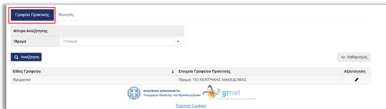
Εικόνα 5.2 – Επιλογή φίλτρων
