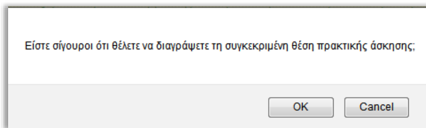
Εικόνα 3.6.2 – Επιβεβαίωση Διαγραφής
