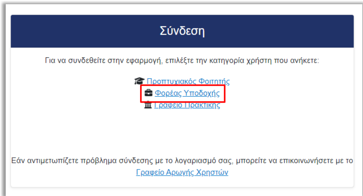
Εικόνα 1.1 – Σύνδεση
