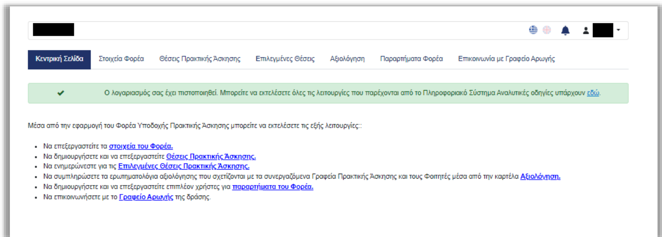
Εικόνα 1.3 – Κεντρική Σελίδα
